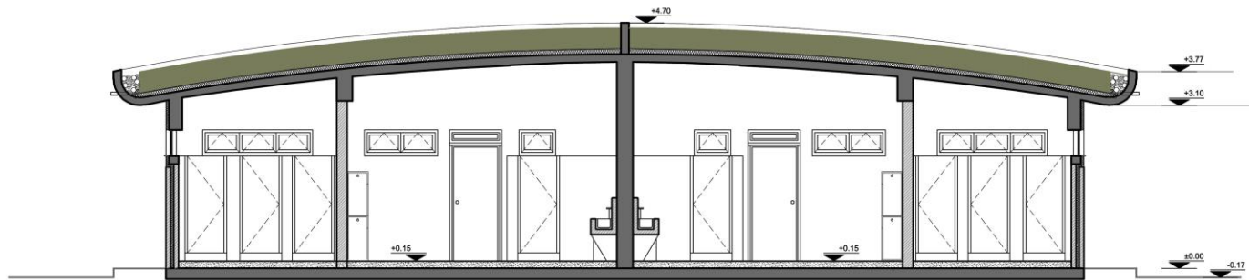
ΤΟΜΗ A-A
