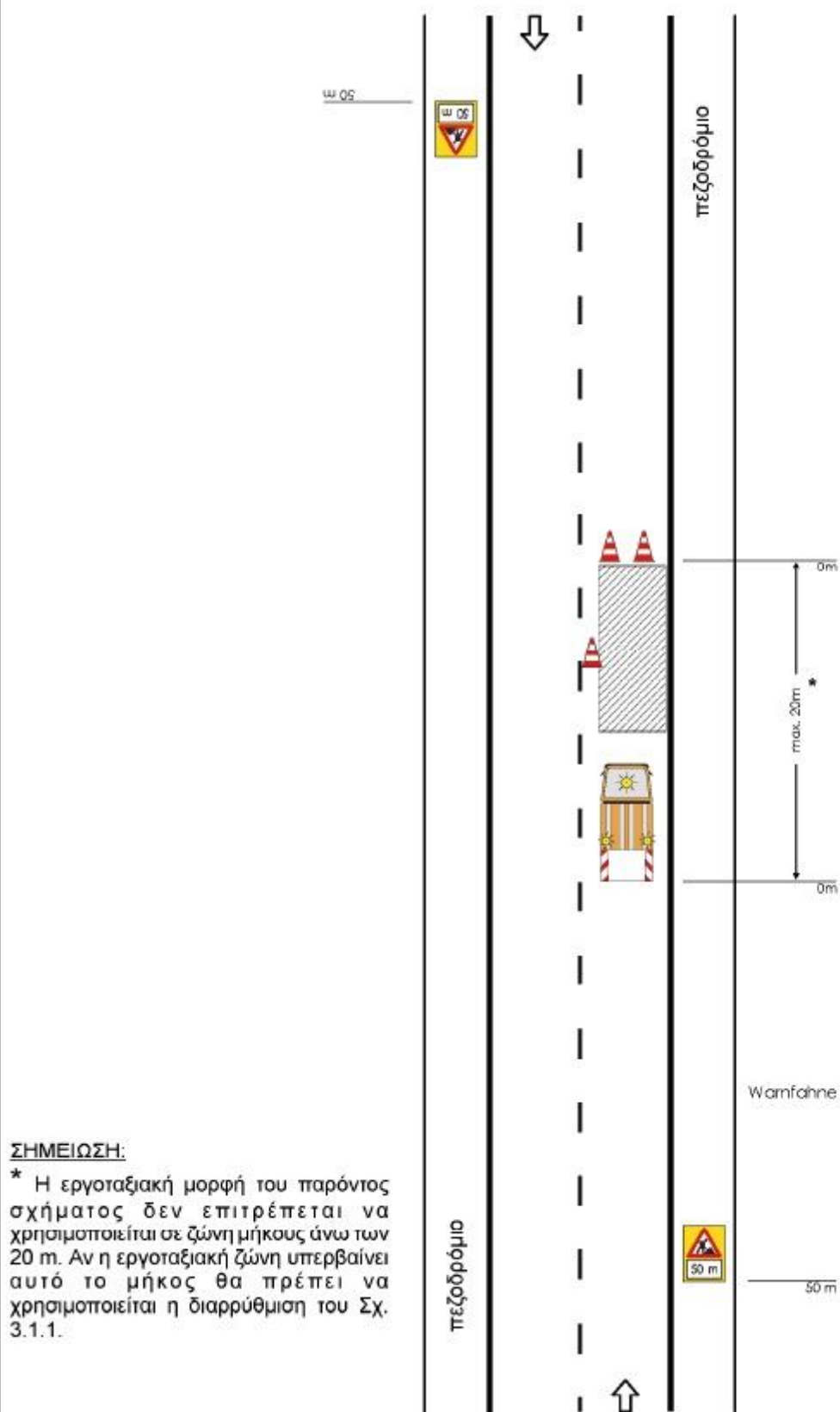
Σχέδιο 3.2.1 : Αποκλεισμός λωρίδας σε κύρια αστική οδό.
