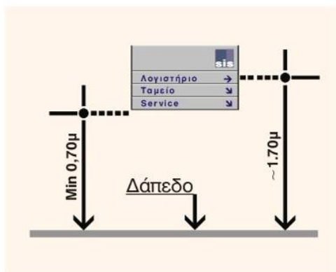
1. Επίτοιχη πινακίδα.
