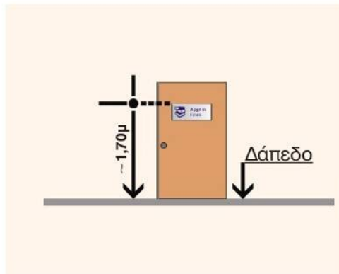
6. Πινακίδα επίθυρη.
