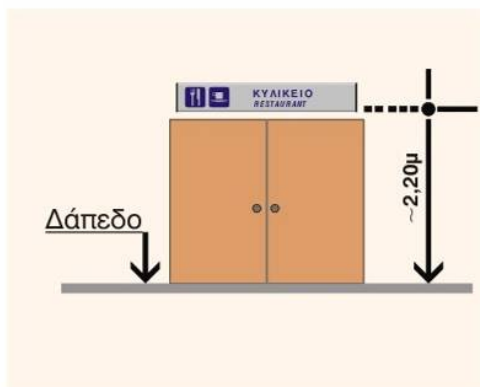
2. Επίτοιχη πινακίδα πάνω απο θύρα.
