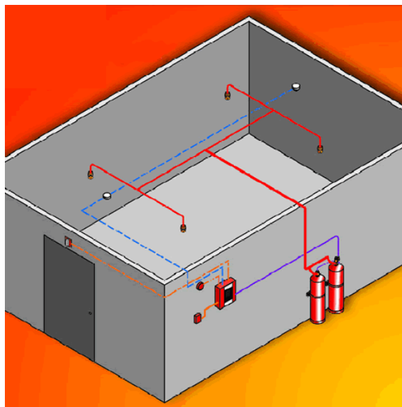
ΤΥΠΙΚΗ ΔΙΑΤΑΞΗ ΕΓΚΑΤΑΣΤΑΣΗΣ (ΕΙΚ.2)
