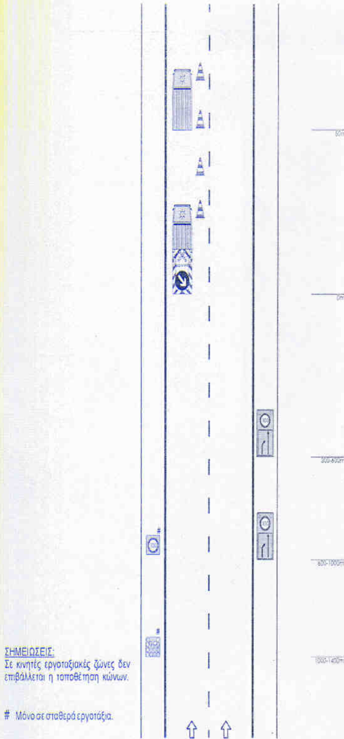
Σχέδιο 1.2.2: Κλείσιμο αριστερής λωρίδας.
