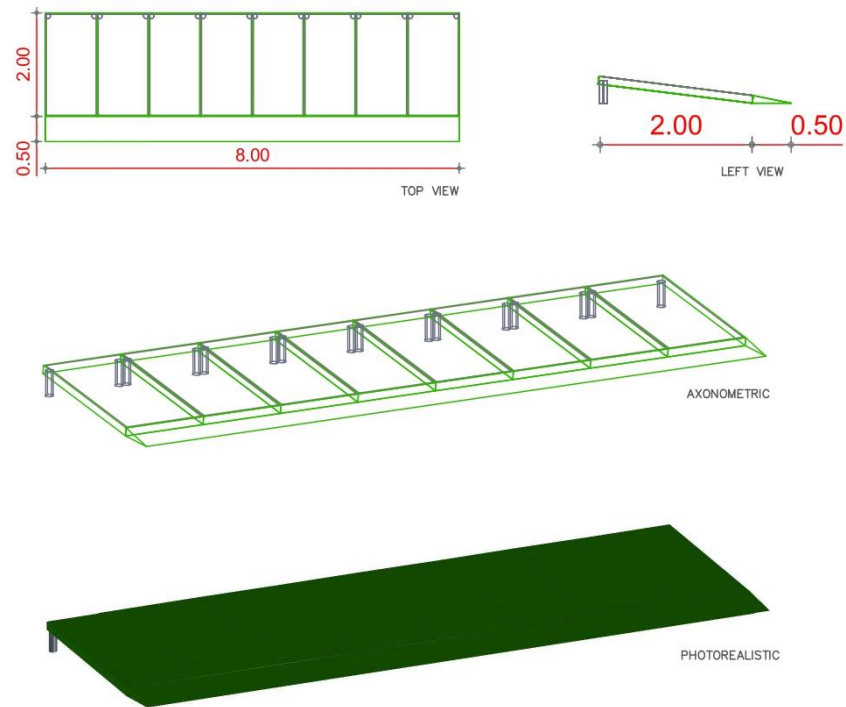
ΣΧ.6γ ΡΑΜΠΑ ΕΙΣΟΔΟΥ ΑΘΛΗΤΩΝ/ΑΥΤ. ΚΑΛΛΙΜΑΡΜΑΡΟ
