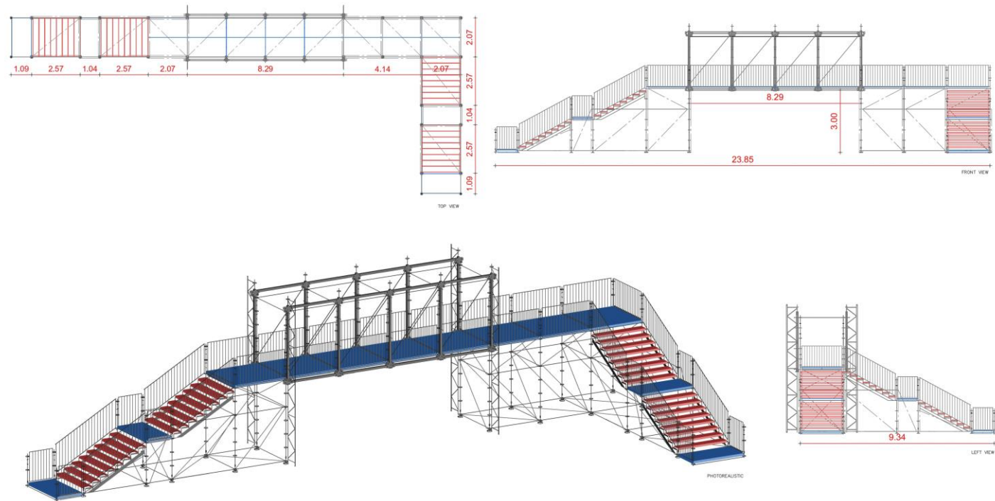
ΣΧ.2 ΠΕΖΟΓΕΦΥΡΑ ΗΡ. ΑΤΤΙΚΟΥ - Β. ΚΩΝ/ΝΟΥ
