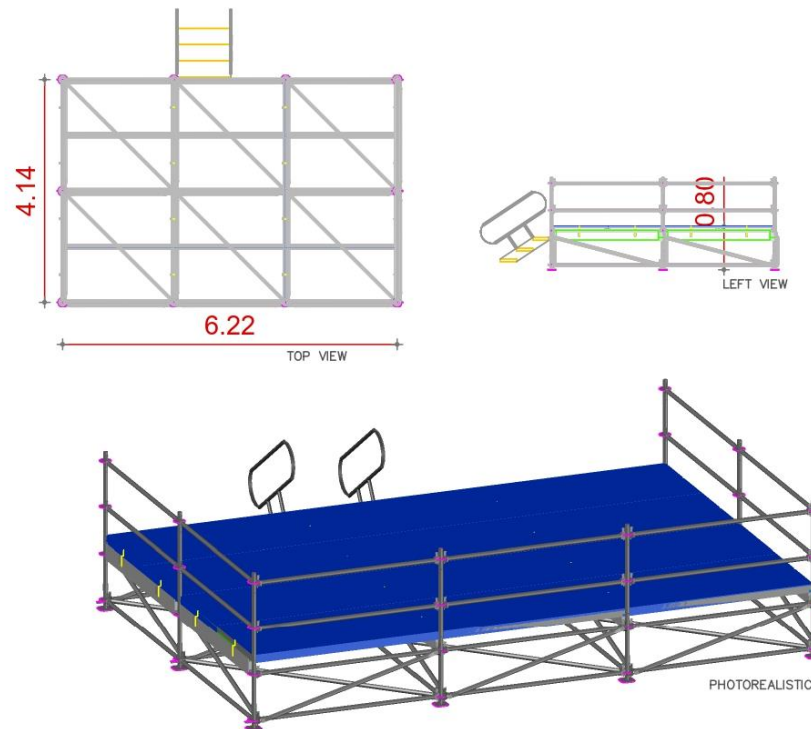
ΣΧ.11 ΕΞΕΔΡΑ ΕΚΚΙΝΗΣΗΣ 5&10 ΧΛΜ Λ. ΑΜΑΛΙΑΣ
