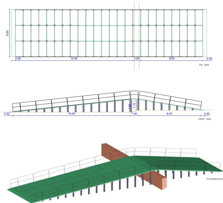
ΣΧ.7α ΡΑΜΠΑ ΕΞΟΔΟΥ ΑΘΛΗΤΩΝ ΜΑΡΑΘΩΝΑΣ
