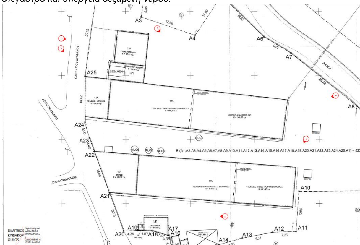
Απόσπασμα τοπογραφικού διαγράμματος της εγκατάστασης
