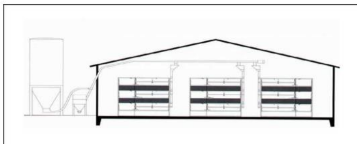
Σχηματική τομή πτηνοτροφικού θαλάμου
