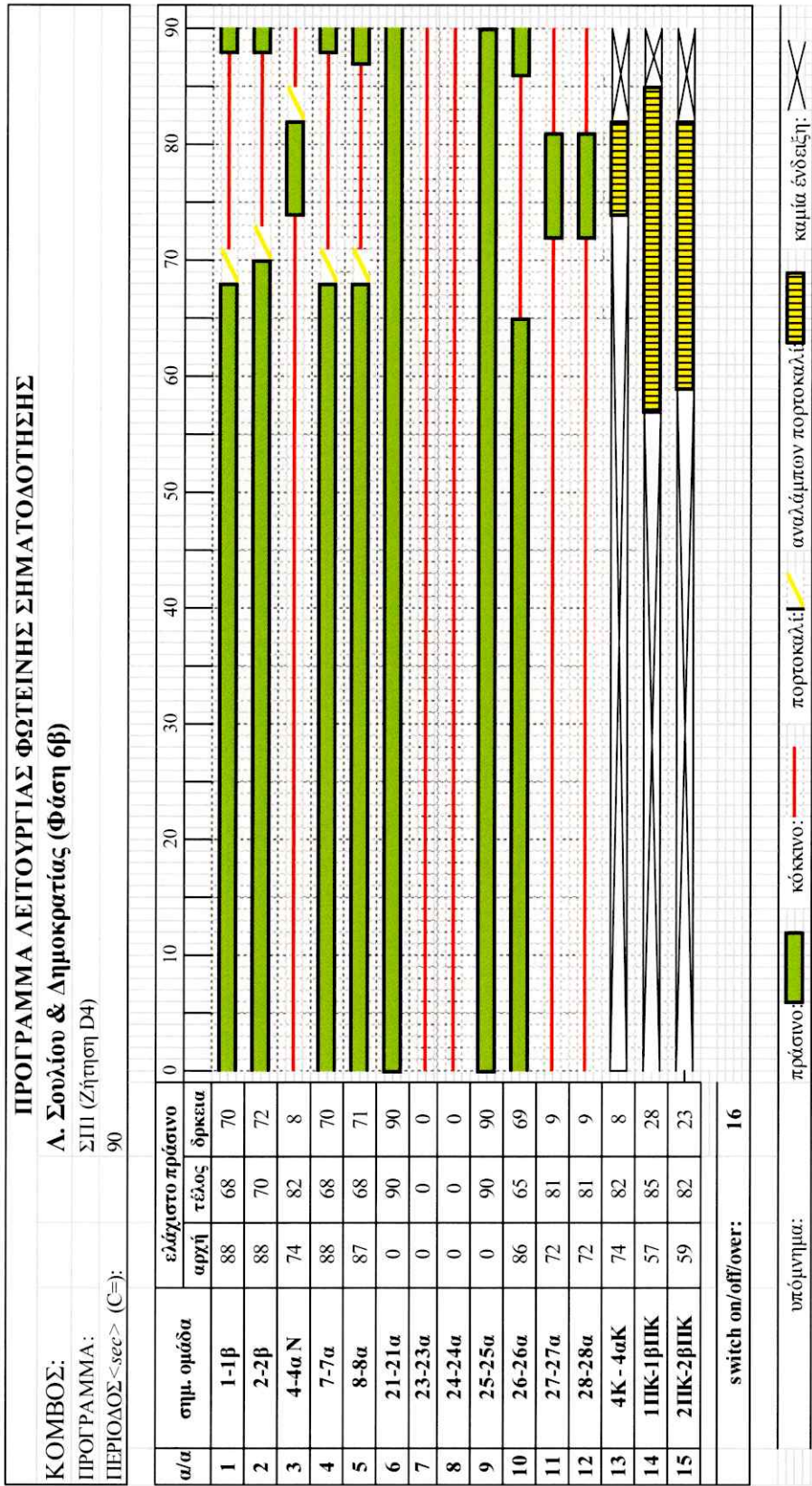
Εικόνα 3. Σηματοδοτικό Πρόγραμμα ΣΠ1 (Ζήτηση D4)
