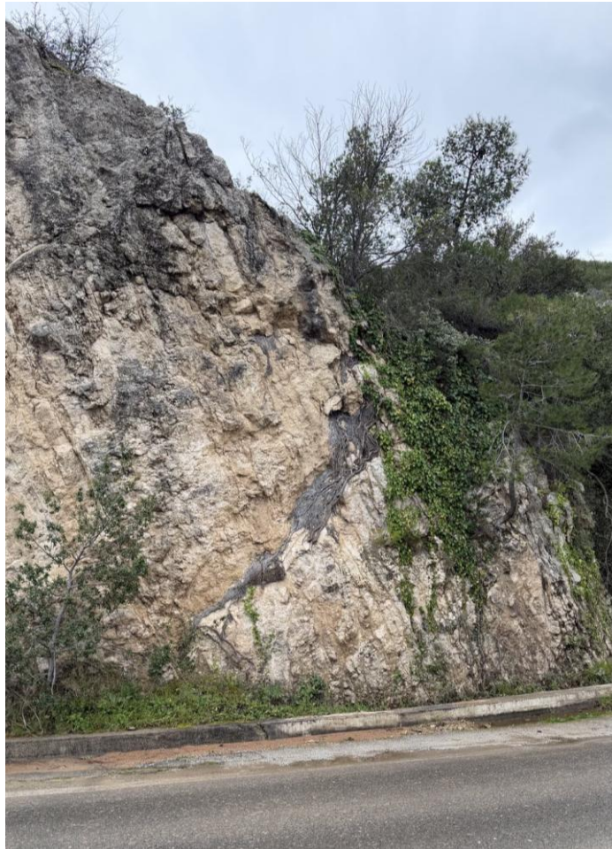
Εικόνα 4. Απεικόνιση βλαβών-αστάθεια πρανών
